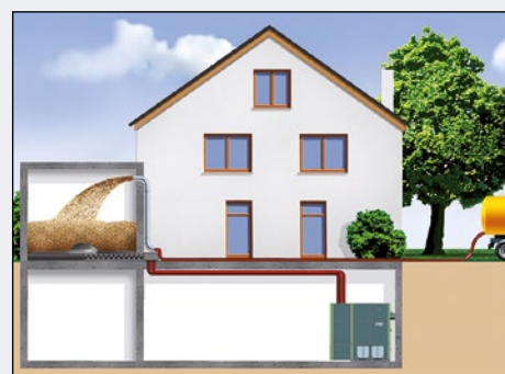
Silo de stockage éloigné de la chaufferie, transport des granulés par système d'aspiration HDG
