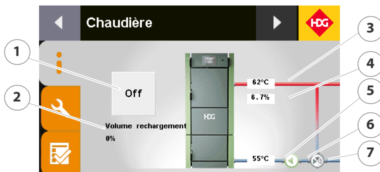
Figure 8/3 - Page d'information de la chaudière
