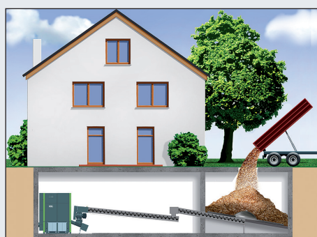
Transport du combustible à partir du silo de stockage situé à distance grâce à une deuxième vis d'alimentation
